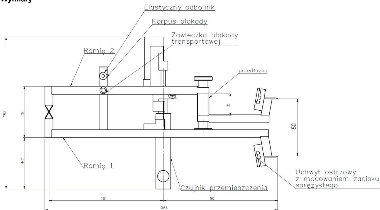
Rys. 1 Elementy składowe ekstensometru z zaznaczeniem gabarytów i wymiarów istotnych z punktu widzenia własności użytkowych (przedstawiona konfiguracja bez płytek dystansowych, o wartości bazy pomiarowej 50mm).
